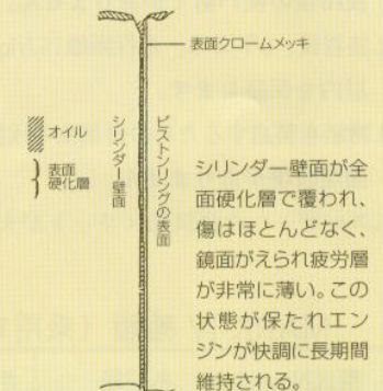
図III. PECS 装着車壁面状態図 (7000~10000km走行時)
