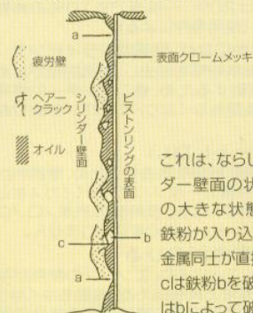
図I. シリンダー対ピストンリングの一次摩耗状態 (ならし運転中の初期現象)
